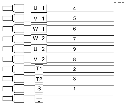
Σύνδεση πίνακα
