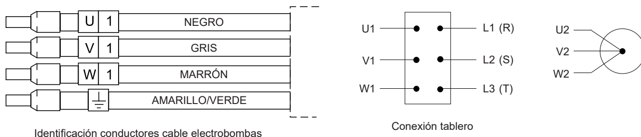
Identificación conductores cable electrobombas
